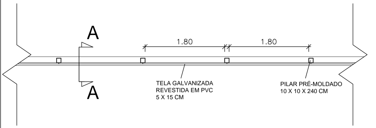
PLANTA BAIXA - DET. DO MURO ESCALA 1/50
