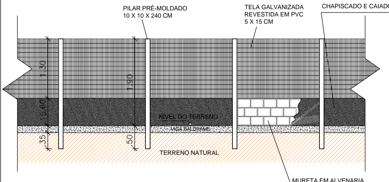
CORTE AA - DET. DO MURO ESCALA 1/50
